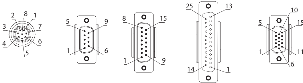
C2: M12 plug (male) C3: D-SUB 9 (male) C4: D-SUB 15 (male) C5: D-SUB 25 (female) C6: D-SUB 15 HD (male)
